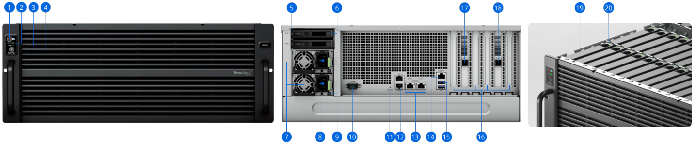
前面板
